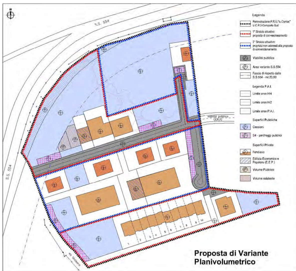
Fig. 6 - Planivolumetrico di progetto
